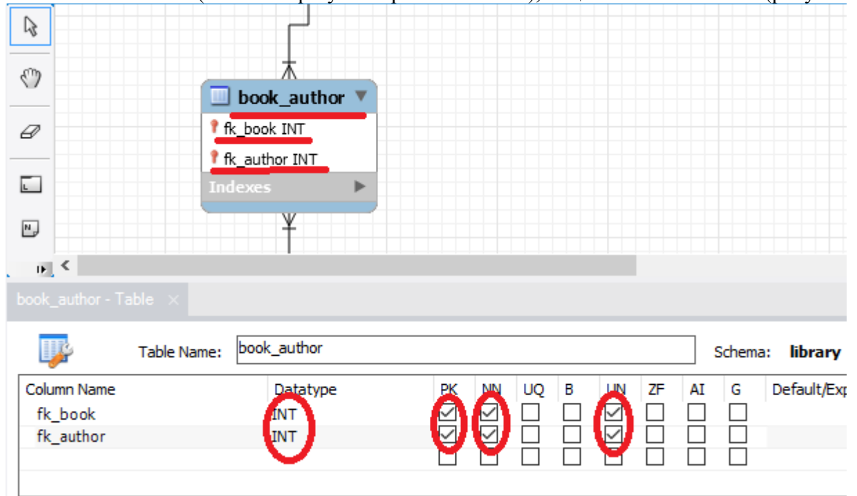
Рисунок 7 – Связывание таблиц N:N
