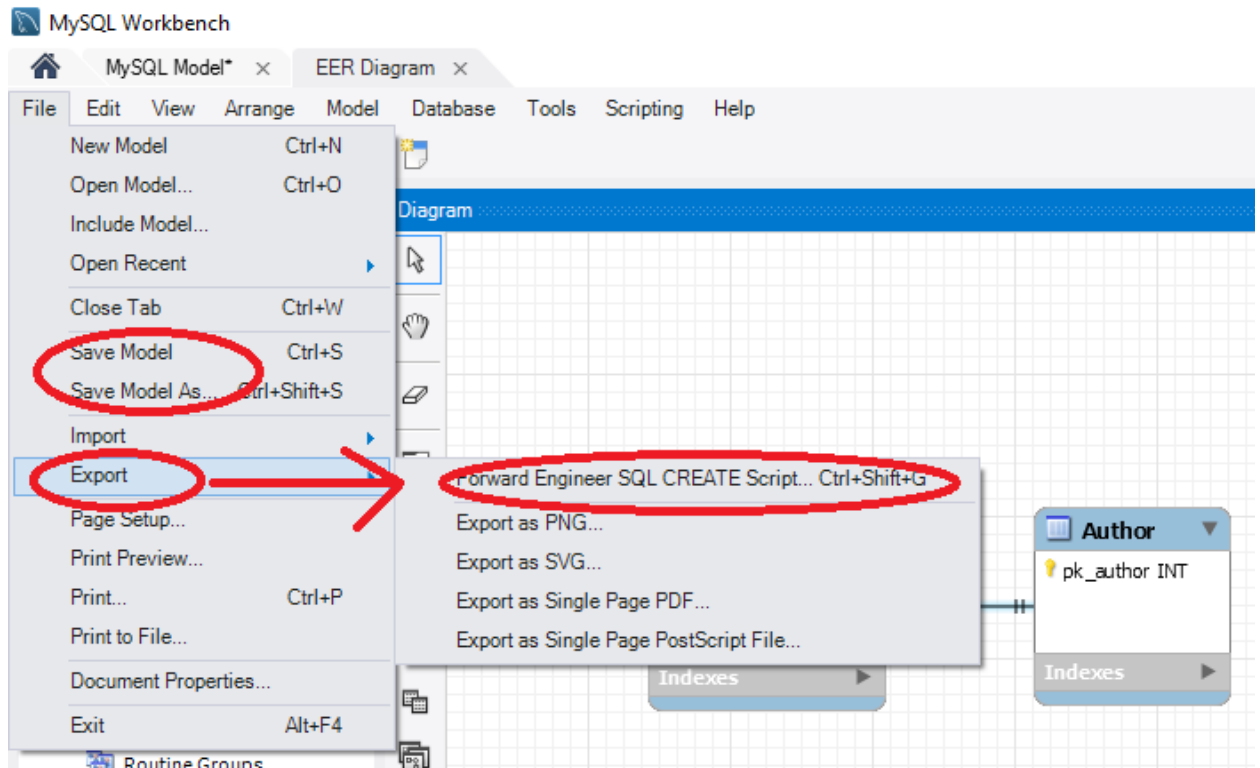
Рисунок 10 – Генерация скрипта
